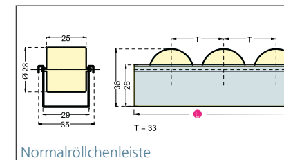
Normalröllchenleiste
